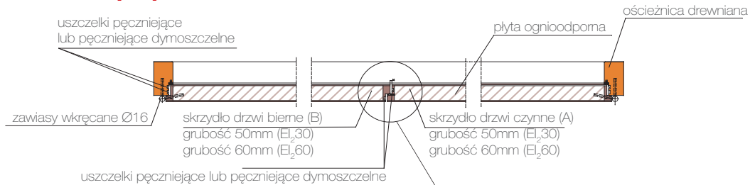
DRZWI DWUSKRZYDŁOWE PRZECIWPÓŻAROWE EI 1,30 , EI 1,60 PRZEKRÓJ POPRZECZNY
