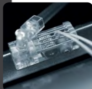
Mechanizm samoblokujący (PATENT) Pokrętko PCV Wieszak bezinwazyjny
