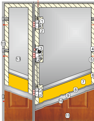
KMT PLUS 54 - dostawka nie otwierana
