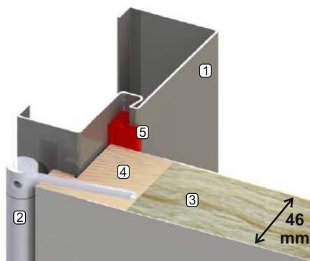
KMT P.poż. EI,30
