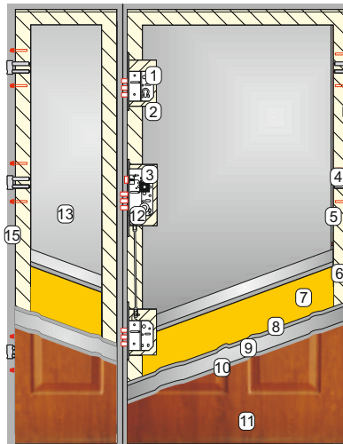
KMT PLUS 75 - dostawka nie otwierana
