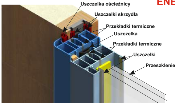
SKRZYDŁO KMT PLUS 75 passive PROFIL OŚCIEŻNICY ENERGY 90 + PROFIL NAŚWIETLA
