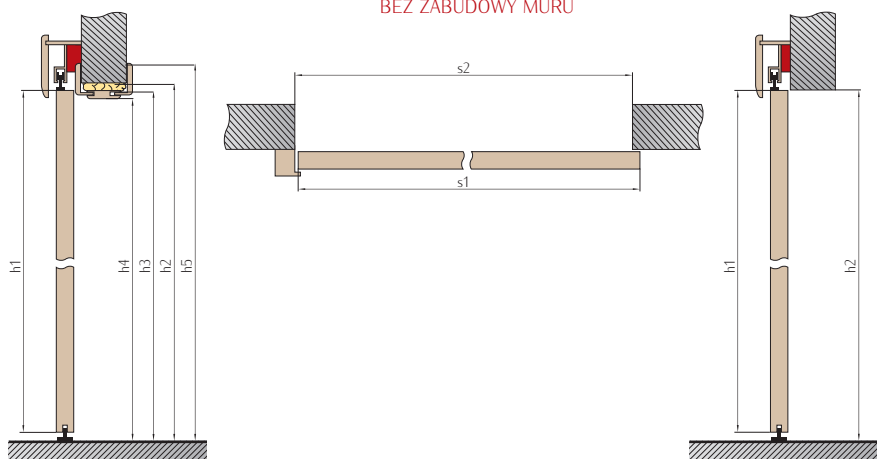
SYSTEM PRZESUWNY BEZ ZABUDOWY MURU
