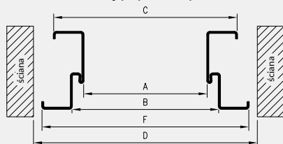
Przekrój poprzeczny
