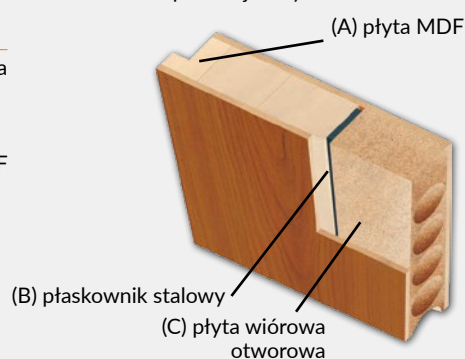
przekrój skrzydła ENTER natura
