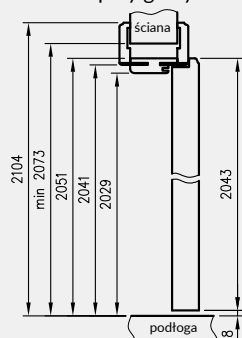
Przekrój pionowy drzwi przylgowych OR
