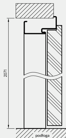
Przekrój pionowy alternatywny sposób montażu
