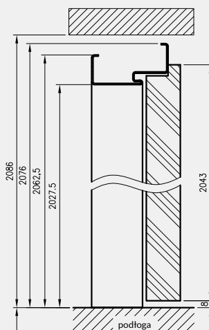
Przekrój poprzeczny alternatywny sposób montażu
