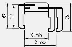
Przekrój TUN Natura z ką. N63
