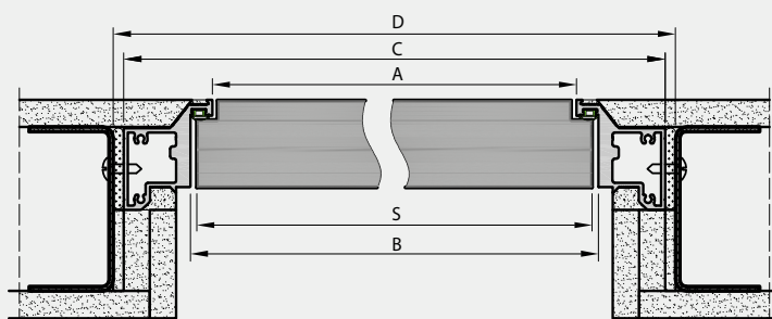
Przekrój poprzeczny drzwi Sara Eco (montaż w ścianie G-K)
