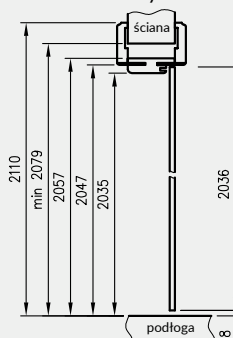
Przekrój pionowy drzwi szklanych ORC
