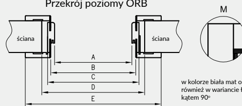
Przekrój poziomy ORB
