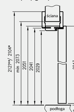
Przekrój pionowy drzwi przyłgowych z OR
