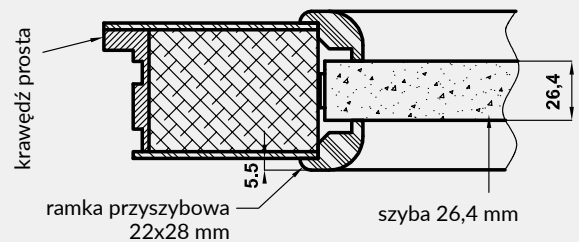
konstrukcja skrzydeł przeciwpożarowych Olimp EI60
