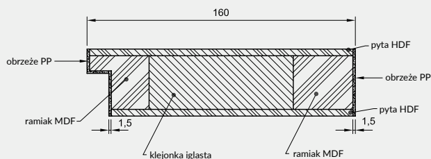
PRZEKRÓJ RAMIAKA PIONOWEGO
