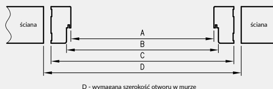
Przekrój poziomy ościeżnicy w murze
