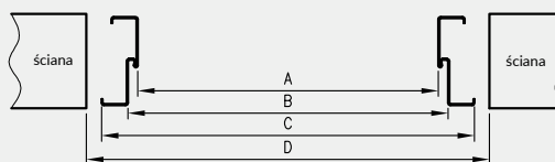
Przekrój poziomy ościeżnicy w murze
