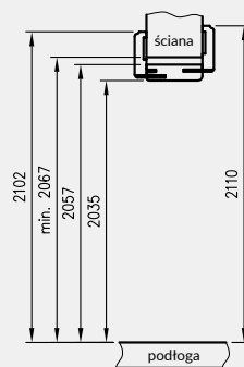
Przekrój pionowy tunelu regulowanego z ką. K63 lub N63
