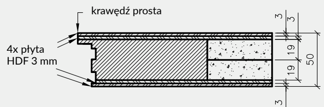
Skrzydło przylgowe przeciwpożarowe Athos EI 30
