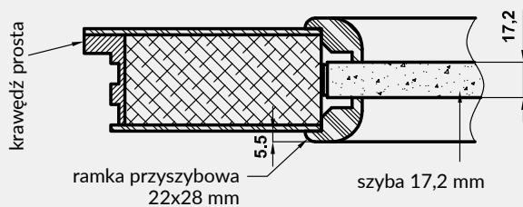
konstrukcja skrzydeł przeciwpożarowych Olimp EI30
