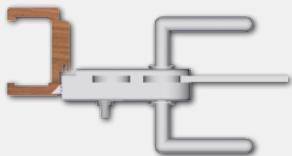
rys. 1. drzwi prawe / blokada na zewnątrz
