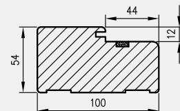
Przekrój poziomy ościeżnicy w murze
