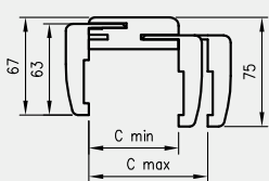
Przekrój TUN z ką. T80
