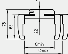
Przekrój OR/ORC Natura z ką. N63
