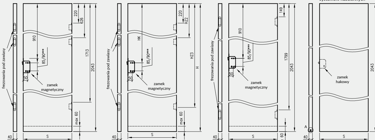
Skrzydła bezprzylgowe rozwiernie Standard 10, Modern, Plus
