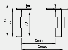
Przekrój OR z ką. T80
