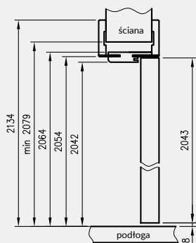
Przekrój pionowy drzwi bezprzylgowych ORB
