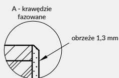
Przekrój ramienia skrzydła bezprzylgowego
