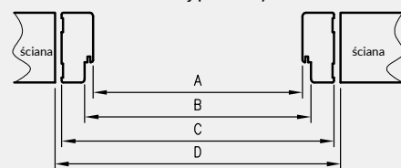
Przekrój poziomy
