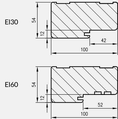
Przekrój ościeżnicy drewnianej p.poż. do skrzydeł OLIMP
