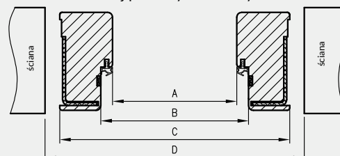
Przekrój poziomy ościeżnicy w murze
