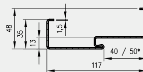
Przekrój ościeżnicy metalowej p.poż. do skrzydeł OLIMP
