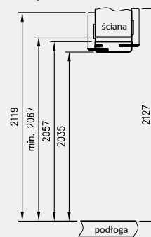
Przekrój pionowy tunelu regulowanego z ką. T80
