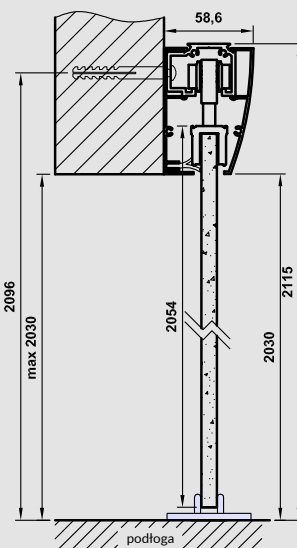
A - A przekrój pionowy systemu Spazio TO
