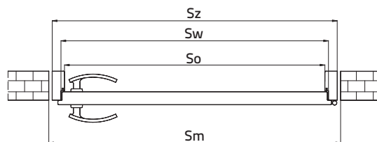
WYMIARY OŚCIEŻNIC STAŁYCH O/MU DO DRZWI JEDNOSKRZYDŁOWYCH
