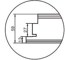
Przekrój skrzydła
