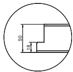
Przekrój skrzydła EI 2 30 F1, F2
