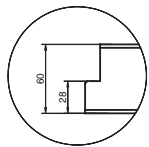
Przekrój skrzydła EI 2 60 F3, F4
