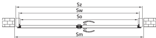
WYMIARY OŚCIEŻNIC STAŁYCH MU/U DO DRZWI DWUSKRZYDŁOWYCH W TECHNOLOGII STANDARD
