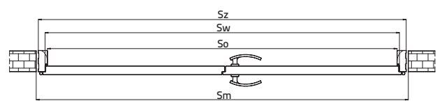
LISTWA OPASOWA O SZEROKOŚCI 60mm (L/MF) / 80mm (L/M8)
