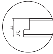
Przekrój skrzydła
