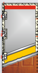
Wzmocnienie pod samozamykacz Dotyczy wykonania wzmocnienia bez zakupu samozamykacza GEZE
