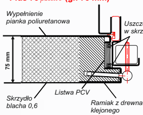
PRZEKRÓJ SKRZYDŁA - Plus 75 passive (gr. 75 mm)
