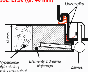
PRZEKRÓJ SKRZYDŁA - P.poż. EI,30 (gr. 46 mm)
