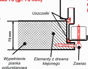
PRZEKRÓJ SKRZYDŁA - Plus 75 (gr. 75 mm)
