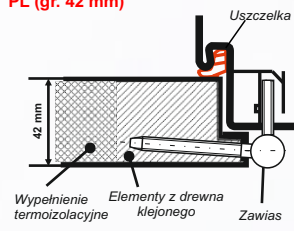
PRZEKRÓJ SKRZYDŁA - PL (gr. 42 mm)
